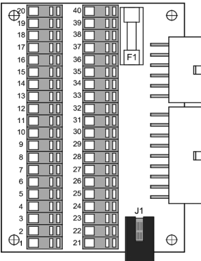
Плата подключений P3
