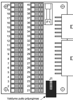
Prijungimo plokštės P3 vaizdas
